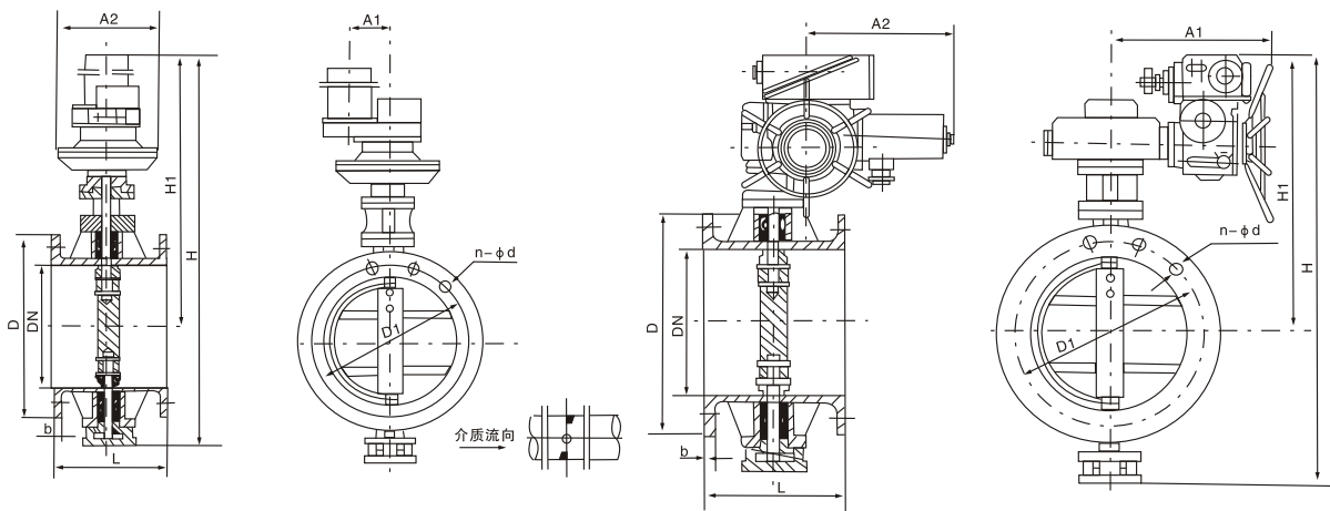
ZD941S-1.5电动式直板式空气蝶阀
