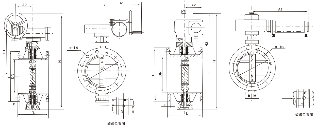
ZD341S-1.5手轮式直板空气蝶阀外形图
